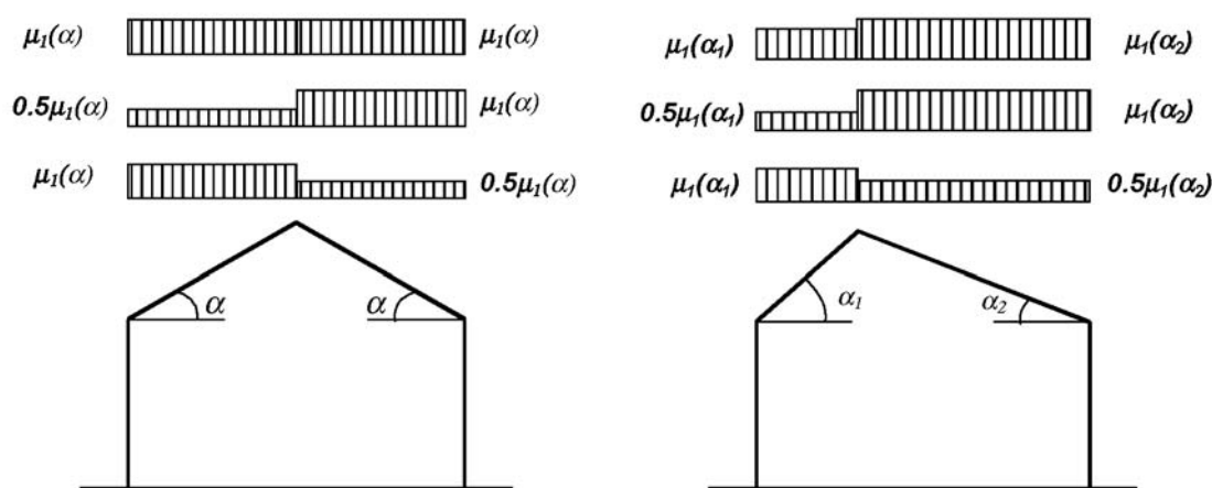
Figura 3.3. Distribuția coeficienților de formă pentru încărcarea din zăpadă pe acoperișurile cu două pante”
